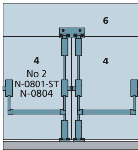
Antipanico verticale standard per doppia porta con sopra luce
