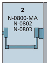
Antipanico orizzontale con bocchetta elettrica e maniglia esterna
