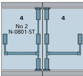
Antipanico verticale Standard per doppia porta
