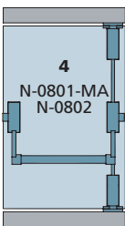
Antipanico verticale standard con maniglia esterna
