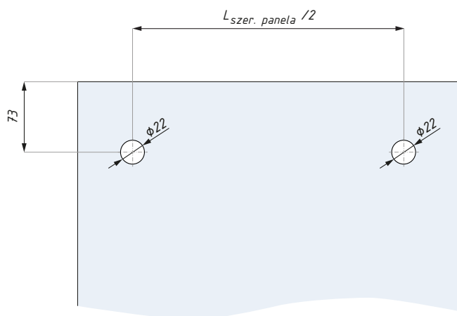
Przygotowanie szkła, panel stały Glass preparation, fixed panel
