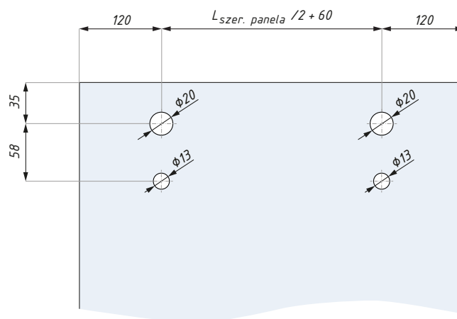
Przygotowanie szkła, panel przesuwny Glass preparation, sliding panel
