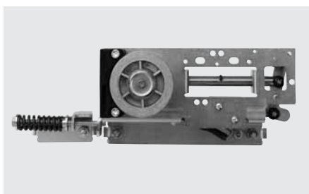
Электромеханический замок на ролике
