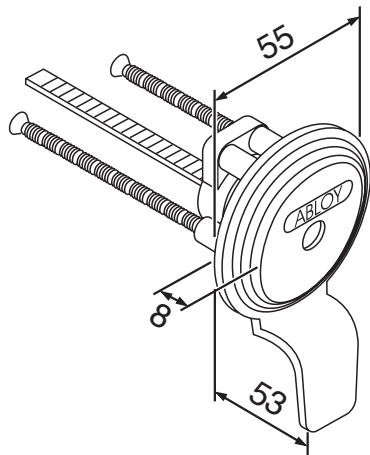
5190, IQ015, IQ115 Pintalukon avainpesä
