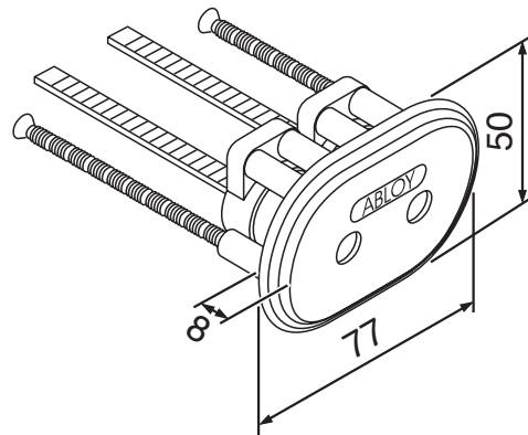
CY026 Pintalukon kaksoisavainpesä
