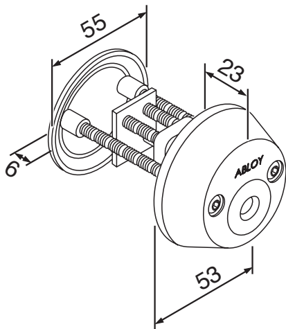
CY034 Sisäpuolinen avainpesä parvekeoviin
