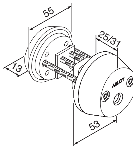
CY061, IQ004, IQ104 Sisäpuolinen avainpesä
