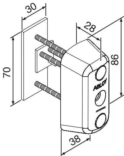
CY063, IQ009, IQ109 Ulkopuolinen avainpesä
