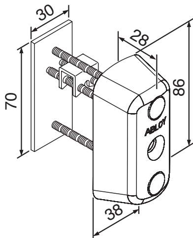
CY047, IQ017, IQ117 Ulkopuolinen avainpesä
