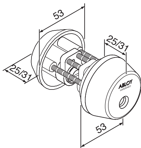
CY062, IQ005, IQ105 Molemminpuoliset avainpesät
