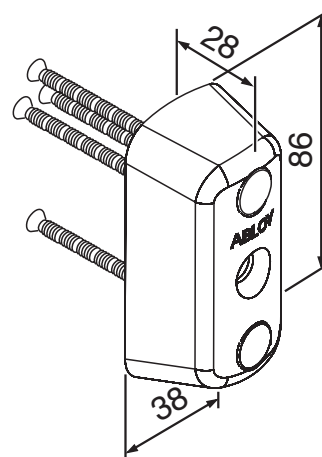
CY052, IQ016, IQ116 Ulkopuolinen avainpesä Avaspuomin ulkopuolinen avainpesä
