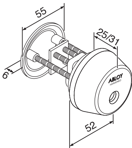
CY060, IQ003, IQ103 Ulkopuolinen avainpesä
