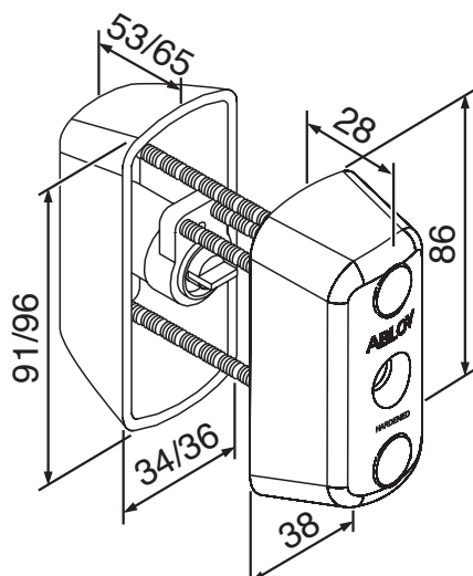
CY065, IQ011, IQ111 Molemminpuoliset avainpesät
