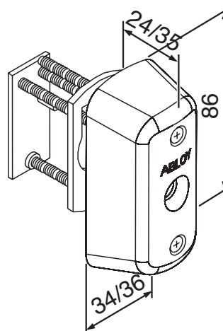
CY064, IQ010, IQ110 Sisäpuolinen avainpesä
