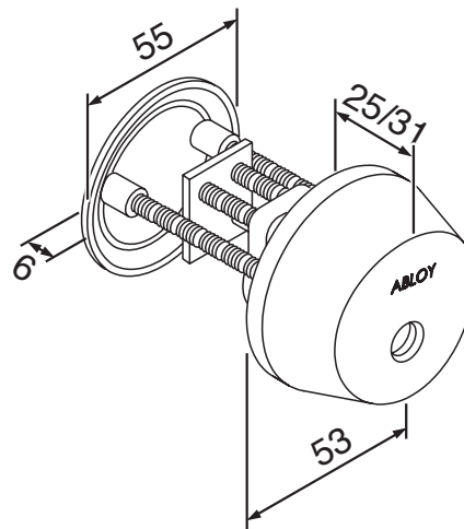
CY037, IQ013, IQ113 Ulkopuolinen avainpesä
